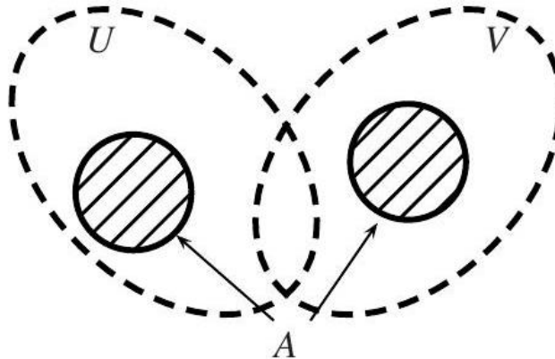
Fig. A.11. A separation of A .
