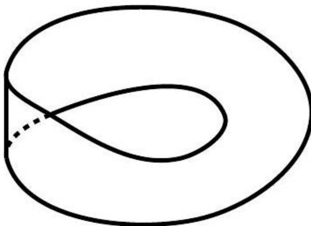
Fig. 21.5. Möbius band.
