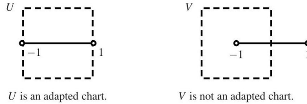
Fig. 9.1.
