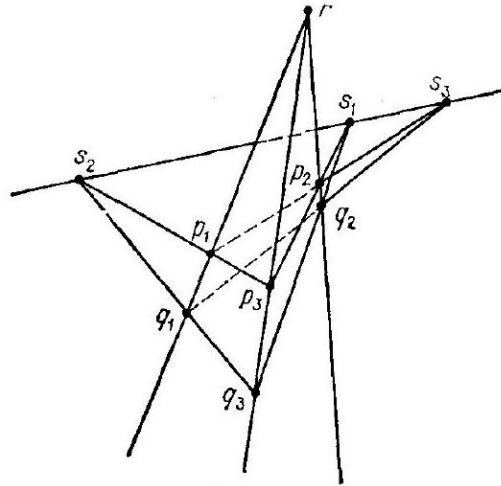
Рис. 8 прямых, сохраняющая отношения инцидентности, транзитивна как на точках, так и на прямых).
