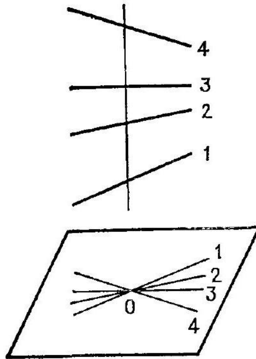
Рис. 7 торое, напомним, определено только на A \setminus \{0\} . Этот график состоит из пар точек с координатами
