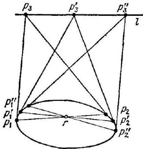
Рис. 4 двойственности точка p_3 отвечает тогда прямой \overline{p_1 p_2} , проходящей через p_1 и p_2 , т. е. проективной оболочке p_1 и p_2 .
